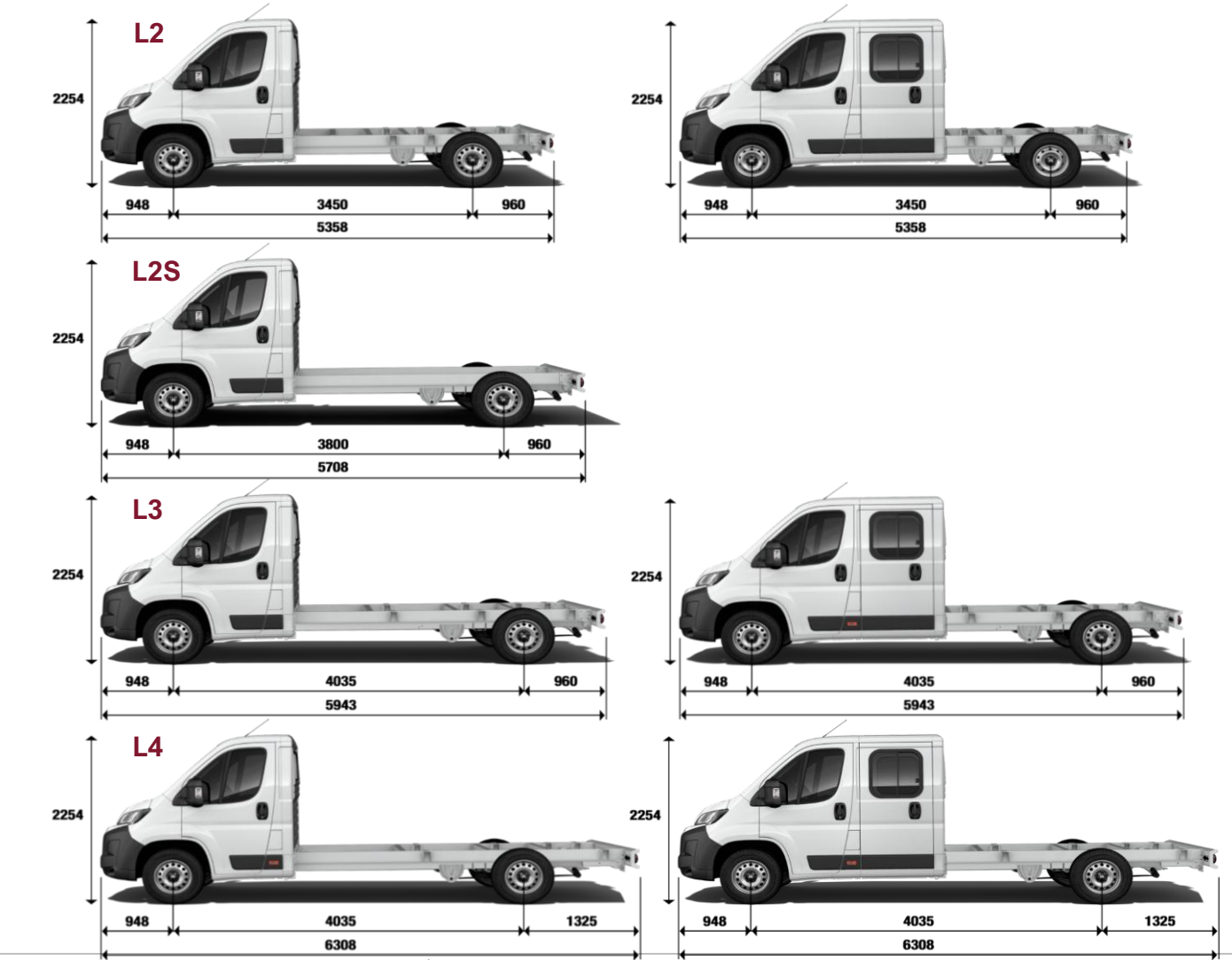
Šasi + kabína
